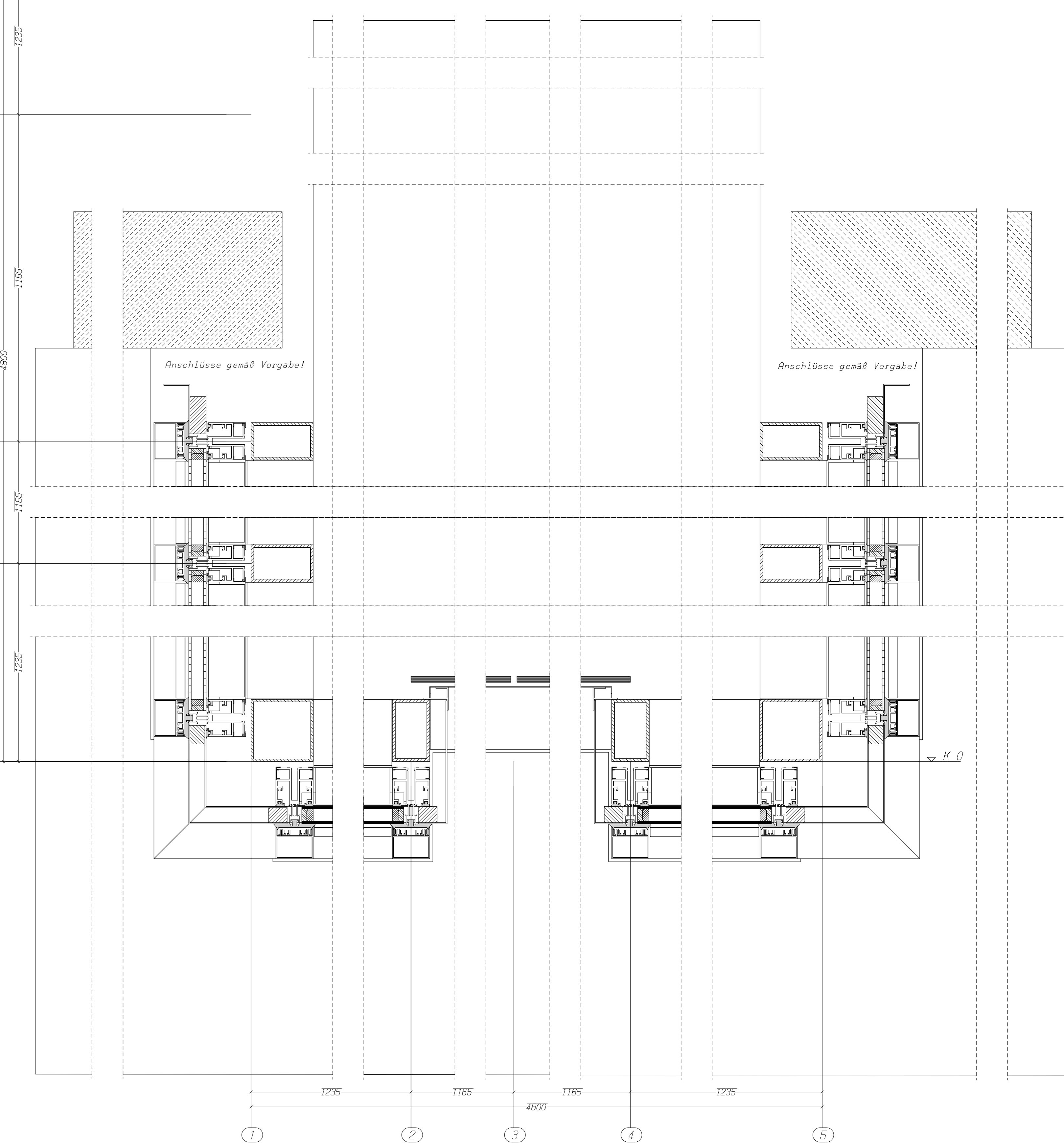
Horizontalschnitt Eingangsturm Eingangsanlage, Maßstab 1:4
