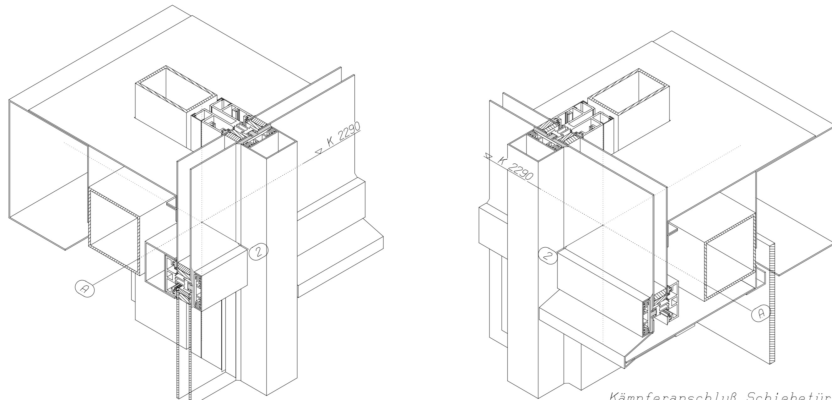
Kämpferanschluß Schiebetür Maßstab 1:4
